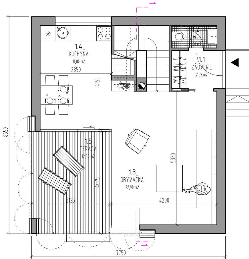
A1/A2 - PÔDORYS PRÍZEMIA
