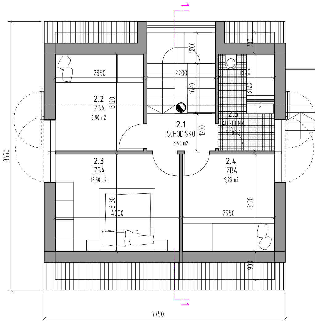
A1/A2 - PÔDORYS PODKROVIA
